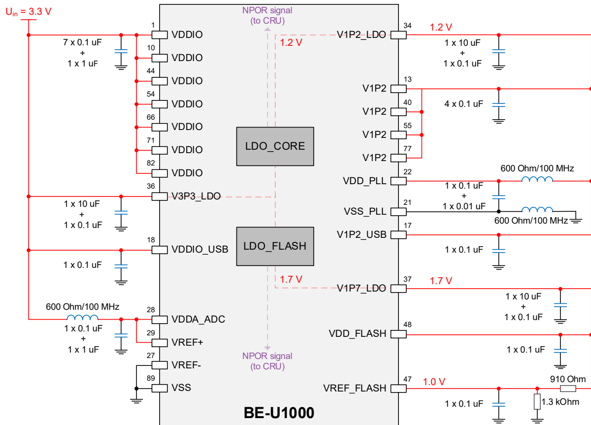
Рисунок 6-1 Схема питания микроконтроллера при использовании LDO
