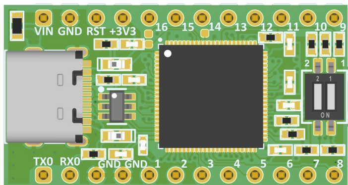
Рисунок 9-1 3D модель платы EVU-LI
