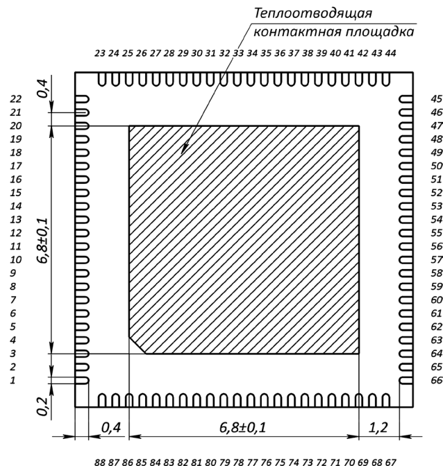
Рисунок 7-4 Габаритные размеры корпуса микроконтроллера (вид снизу)
