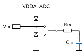
Рисунок 6-3 Эквивалентная схема вывода Vin АЦП
