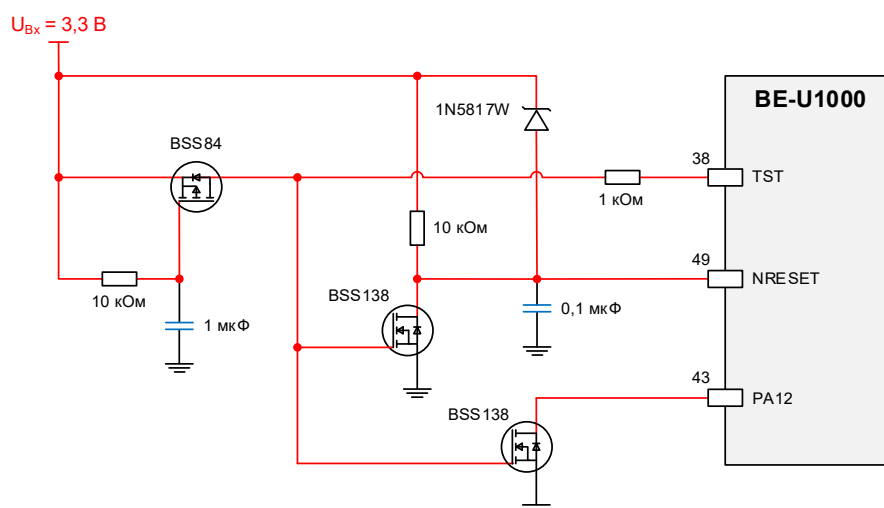
Рисунок 6-2 Пример схемы для запуска микроконтроллера
